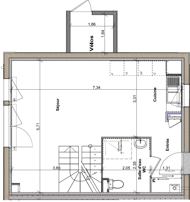
PLAN REZ DE CHAUSSEE Ech: 1/100
