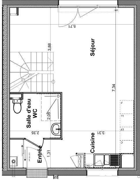
PLAN REZ DE CHAUSSEE Ech: 1/100
