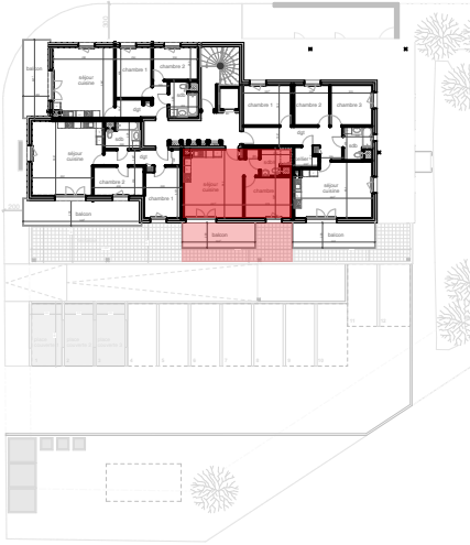
plan de localisation deuxième étage
